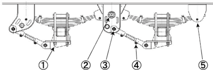
各部の名称と締め付けトルク
