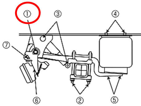
ツーサイドリフトアクスル
